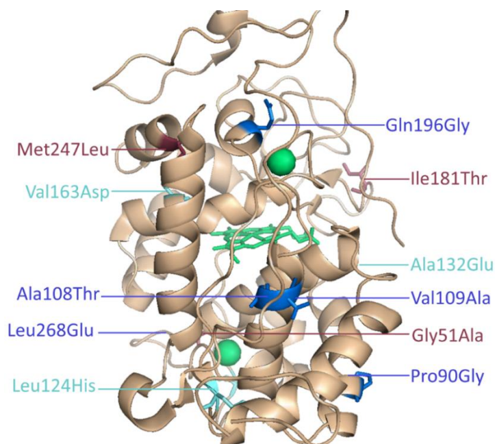
Slika 46. Struktra versatilne peroksidaze sa obeleženim mutiranim pozicijama. Svetlo plavo – MV1; Tamno plavo – MV2; Ljubičasti – MV3
