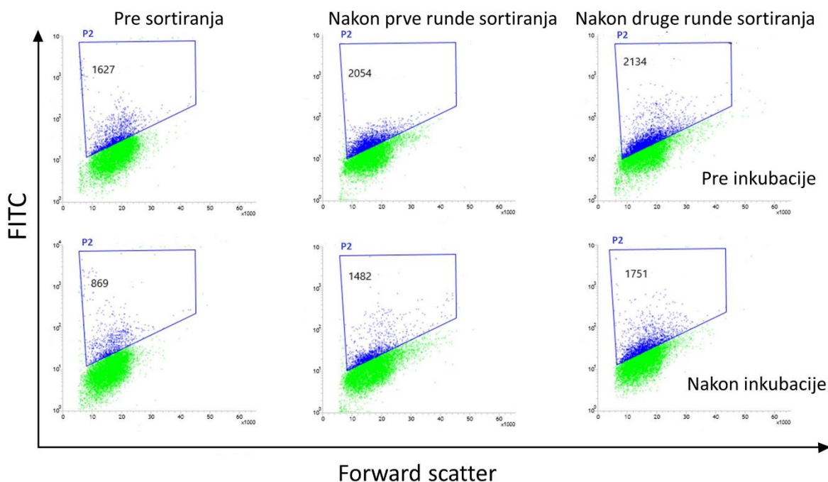
Slika 36. FACS histogrami dobiveni analizom ćelija koje eksprimiraju nasumične biblioteke gena na svojoj površini u toku dve runde sortiranja pre ili nakon inkubacije u 30 mM H_2O_2
