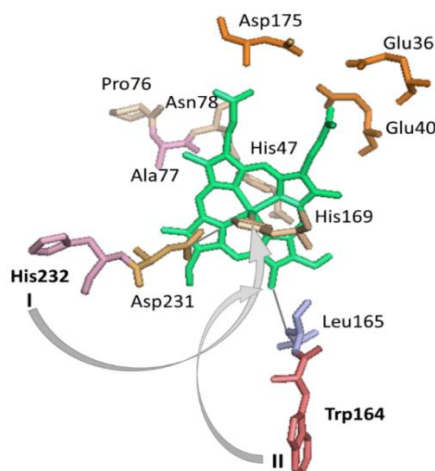
Slika 10. Mogući putevi prenosa elektrona sa supstrata na molekul hema u toku katalitičkog ciklusa versatilne peroksidaze
