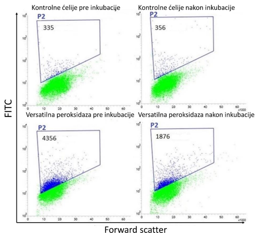
Slika 35. FACS histogrami kontrolnih ćelija i ćelija koje ekspiriraju divlji tip versatilne peroksidaze pre i posle inkubacije u 30 mM H_2O_2
