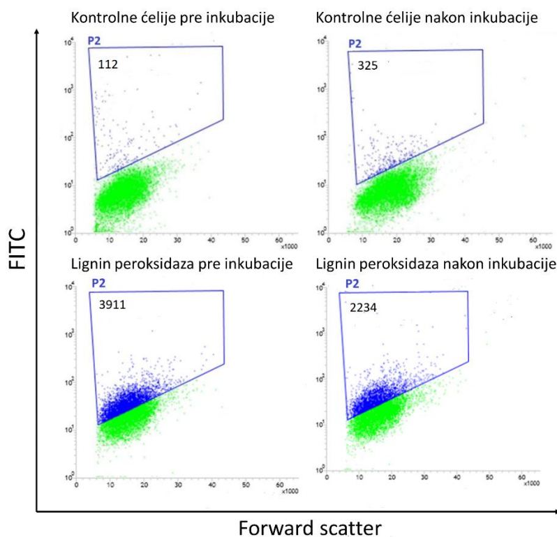
Slika 38. FACS histogrami kontrolnih ćelija i ćelija koje eksprimiraju divlji tip lignin peroksidaze pre i posle inkubacije u 30 mM \text{H}_2\text{O}_2
