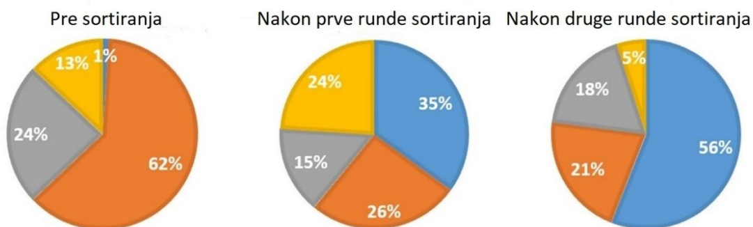
Slika 37. Prikaz broja ćelija koje eksprimiraju varijante versatilne peroksidaze različite oksidativne stabilnosti pre i nakon prve i druge runde sortiranja. Narandžasta boja – ćelije koje eksprimiraju neaktivne mutante VP; Siva boja – ćelije koje eksprimiraju mutante VP niže oksidativne stabilnosti on wtVP; Žuta boja – ćelije koje eksprimiraju varijante enzima sa većom oksidativnom stabilnošću od wtVP.
