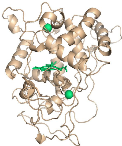
Slika 3. Struktura lignin peroksidaze iz P. chrysosporium H8. Atomske koordinate preuzete su iz PDB fajla 1B82 (Blodig et al., 2001).
