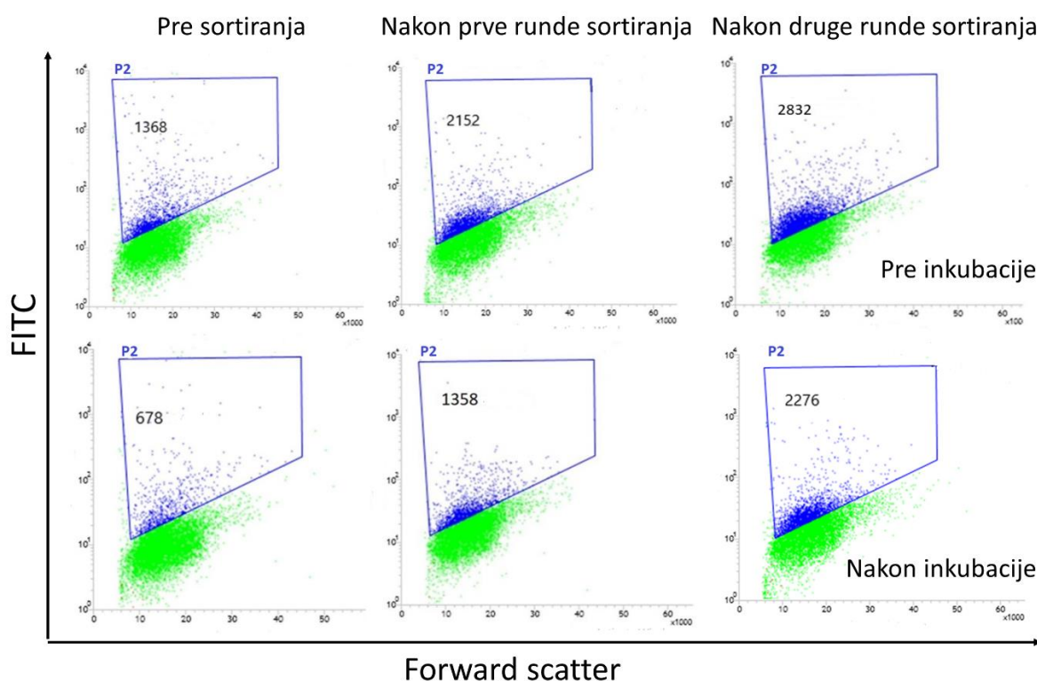
Slika 39. FACS histogrami dobiveni analizom ćelija koje eksprimiraju nasumične biblioteke gena lignin peroksidaze na svojoj površini u toku dve runde sortiranja pre ili nakon inkubacije u 30 mM H 2 O 2
