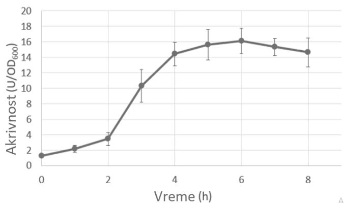
Slika 48. Promena aktivnosti lignin peroksidaze u toku lize ćelija kvasca.
