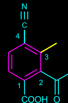
2-ACETIL- 4-CIJANO-3-METIL- -BENZOEVA KISELINA
