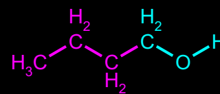
Butan-1-ol
