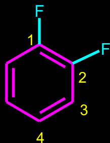
1,2-Difluor-benzen
