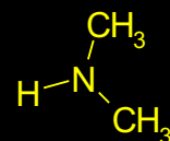
DIMETIL-AMIN
