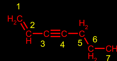
HEPT-1-EN-3-IN
