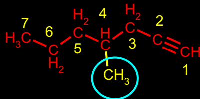
4-METIL-HEPT-1-IN
