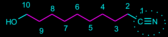
10-HIDROKSI-DEKAN-NITRIL
