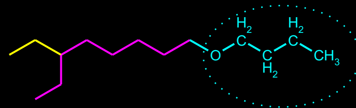
1-Butoksi-6-etil-oktan
