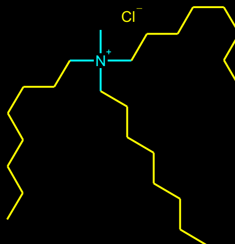
TRI-OKTILL-AMONIJUM METILAMONIJUM HLORID
