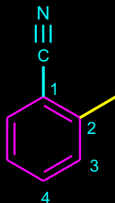
2-METIL- BENZONITRIL
