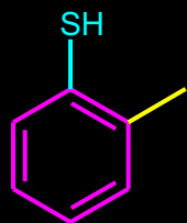
2-METIL-BENZENTIOL
