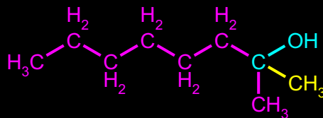
2-Metil-oktan-2-ol
