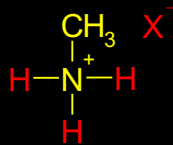
METIL-AMONIUM JON
