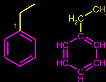
ETIL-BENZEN
