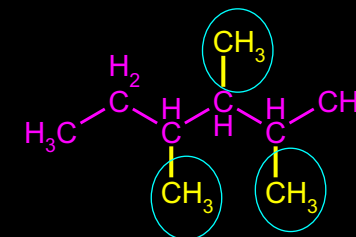
2,3,4-TRI-METIL-HEKSAN
