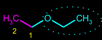
DI-ETIL-ETAR (ETOKSI-ETAN)
