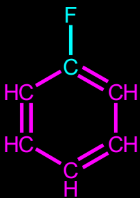
AutoNom Name: Fluoro-benzene
