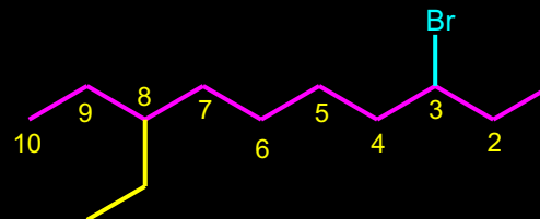
3- BROM-8-ETIL-DEKAN
