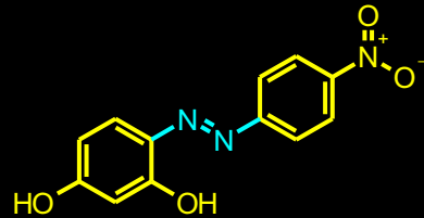
Azo violet
