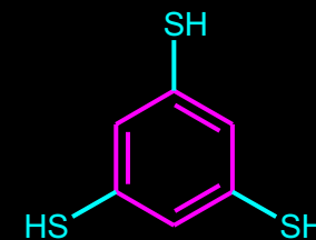
BENZEN-1,3,5-TRITIOL
