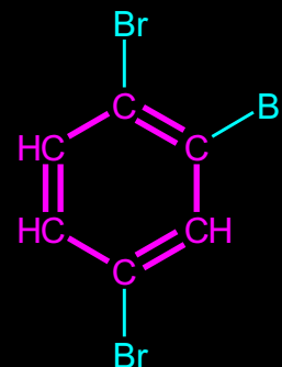
1,2,4-Tribrom-benzen
