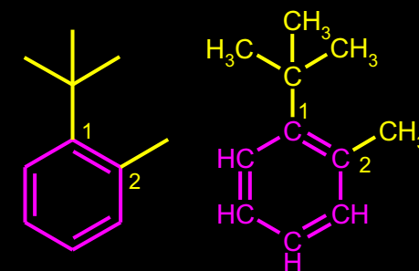
1-terc-BUTIL-2-METIL-BENZEN
