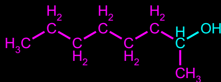
Okatan-2-ol
