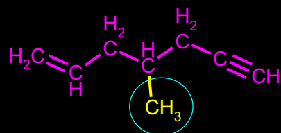
4-METIL-HEPT-1-EN-6-IN
