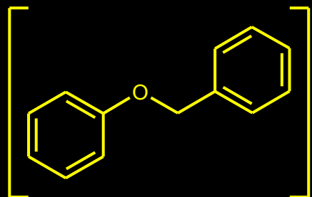
[BENZILOKSI-BENZEN]
