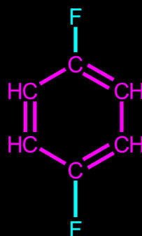
AutoNom Name: 1,4-Difluoro-benzene
