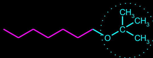
1-terc-Butoksi-heptan
