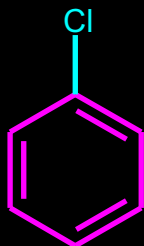
Hlor-benzen
