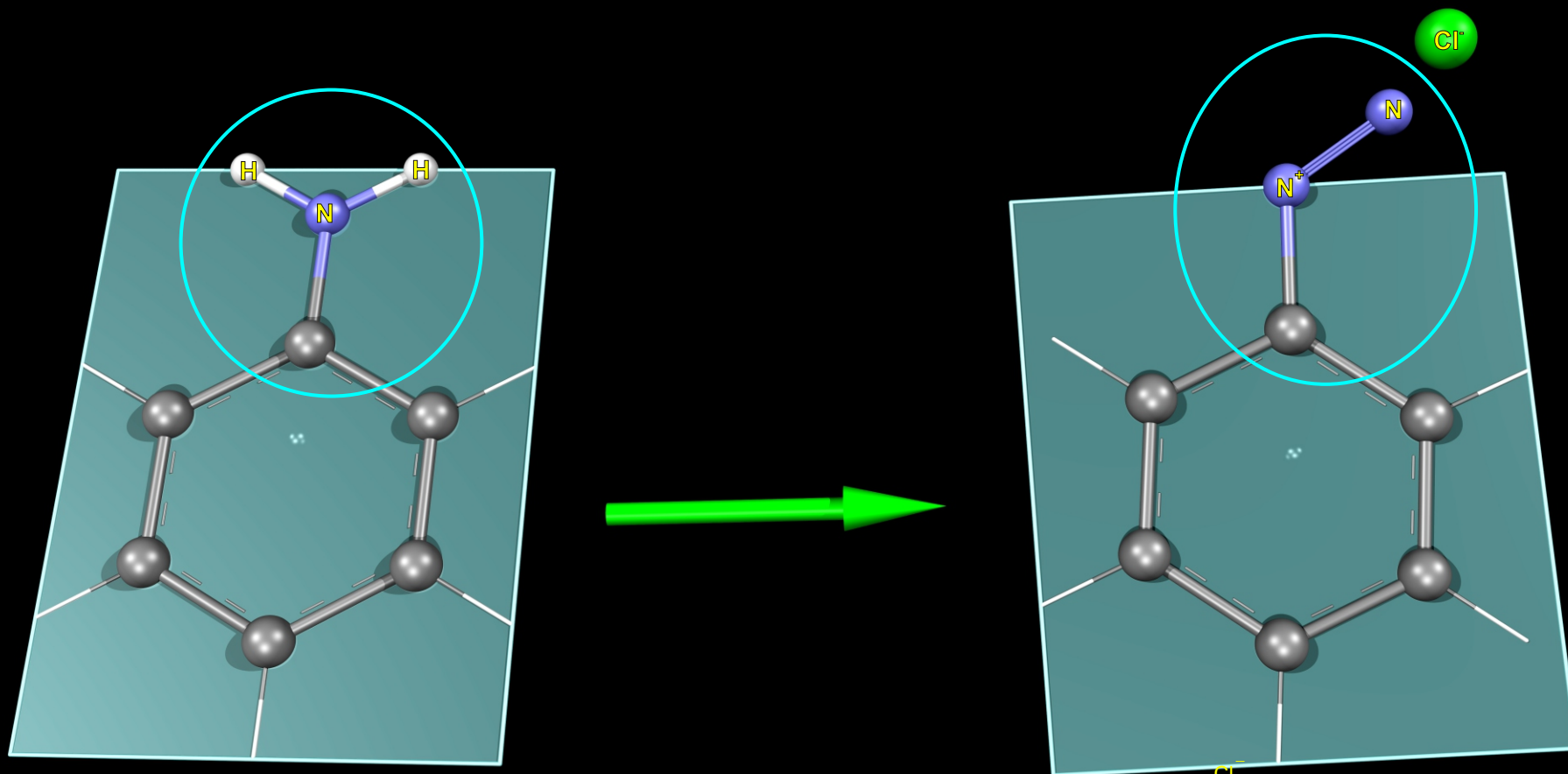
[N+]#Nc1ccccc1.[Cl-] DIJAZONIJUMOVA SO POSTALA IZ ANILINA (BENZEN-DIJAZONIJUM HLORID)
