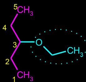
3-ETOKSI-PENTAN)
