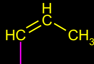
PROPILIDEN
