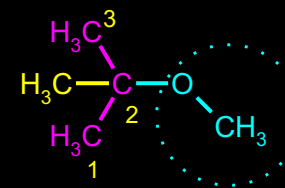
terc-BUTIL-METIL-ETAR (2-METOKSI-2-METIL-PROPAN)
