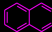
NAFTALEN
