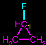
1-FLUOR- CIKLOPROPAN
