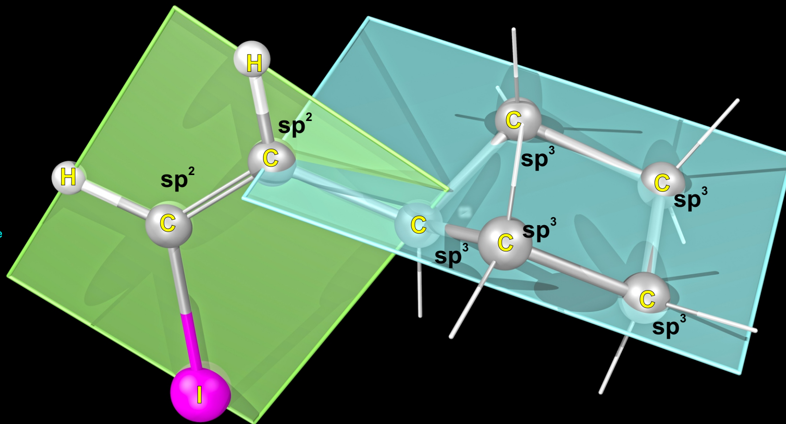
((Z)-2-Iodo-vinyl)-cyclopentane
