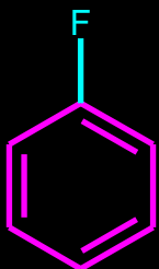
Fluor-benzen
