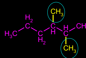
2,3-DIMETIL-HEKSAN
