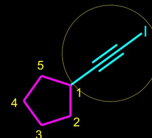
JOD-ETINIL-CIKLOPENTAN
