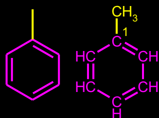
TOLUEN
