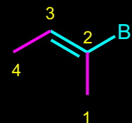
(E)-2-BROM- BUT-2-EN
