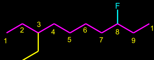
3- ETIL-8-FLUOR-DEKAN
