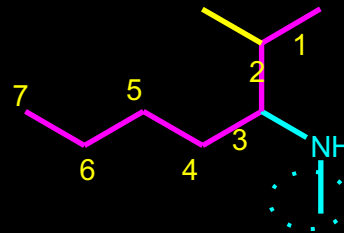
N ,2-dimetil-heptan-3-amin
