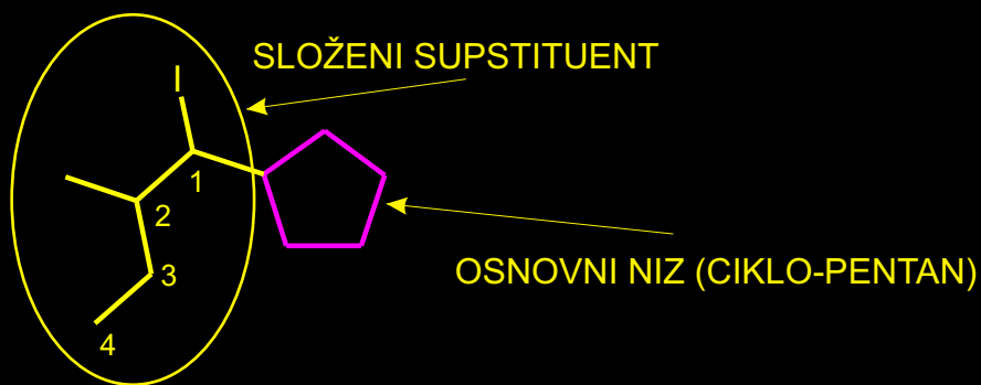
(1-JOD-2-METIL-BUTIL)-CIKLO-PENTAN
