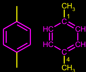
p-KSILEN
