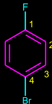
1-Brom-4-fluor-benzen ili p -Brom--fluor-benzen
