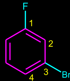
1-Brom-3-fluor-benzen ili m -Brom--fluor-benzen
