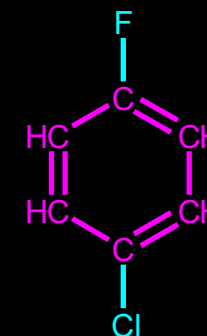
AutoNom Name: 1-Chloro-4-fluoro-benzene
