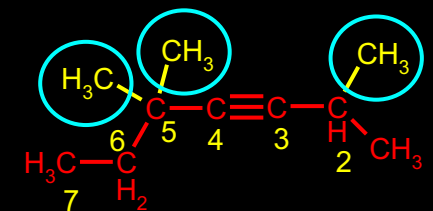
2,5,5-TRI-METIL-HEPT-3-IN
