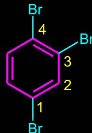
1,3,4-Tribrom-benzen
