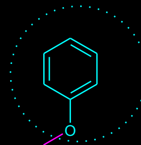
FENOKSI
