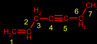
HEPT-1-EN-4-IN
