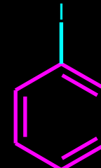
Jod-benzen
