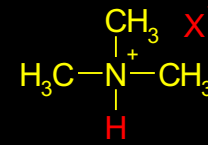
TRIMETIL-AMONIUM JON
