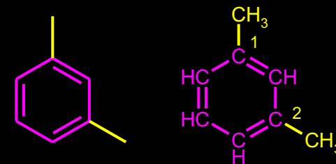
m-KSILEN
