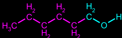
Hexan-1-ol
