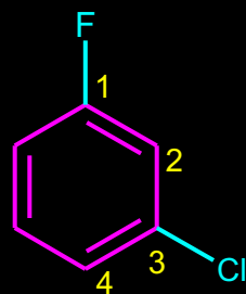
1-Hlor-3-fluor-benzen ili m -Hlor-fluor-benzen
