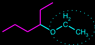
3-Etoksi-hexan
