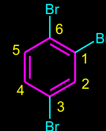
1,3,6-Tribrom-benzen
