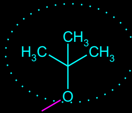
terc-BUTOKSI
