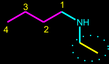
N -etil-butan-1-amin
