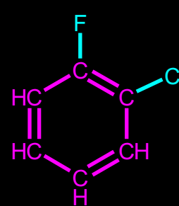
AutoNom Name: 1-Chloro-2-fluoro-benzene
