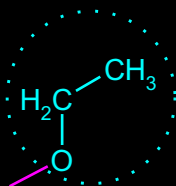
ETOKSI
