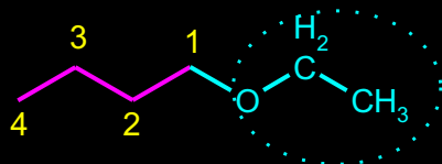
1-Etoksi-butan
