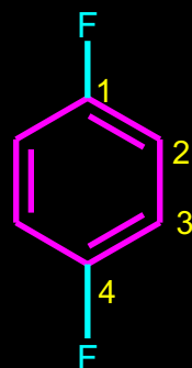
1,4-Difluor-benzen
