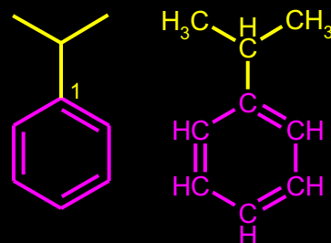
izo-PROPIL-BENZEN
