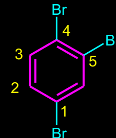
1,4,5-Tribrom-benzen
