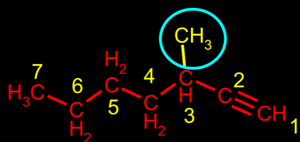
3-METIL-HEPT-1-IN
