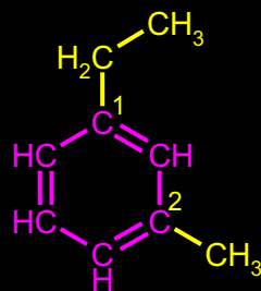
1-ETIL-3-METIL-BENZEN
