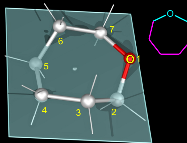
OKSEPAN; OKSACIKLOHEPTAN
