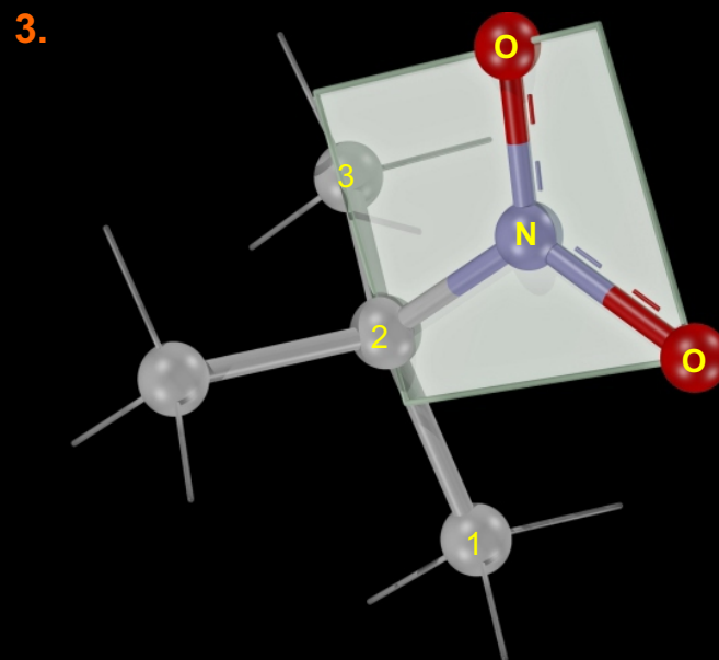
2-METIL-2-NITRO-PROPAN
