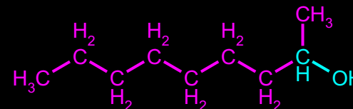
Nonan-2-ol
