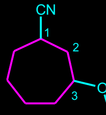
3-METOKSI-CIKLOHEPTAN-KARBONITRIL
