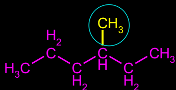
3-METIL-HEKSAN
