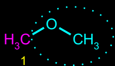
DI-METIL-ETAR (METOKSI-METAN)
