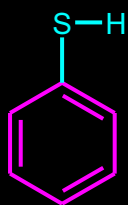
BENZENTIOL
