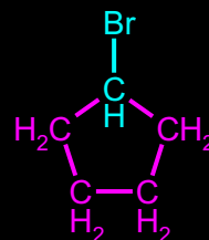
1-BROM-CIKLOPENTAN
