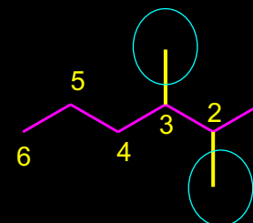
2,3-DIMETIL-HEKSAN
