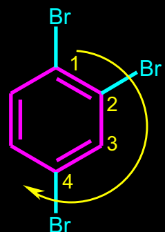
1,2,4-Tribrom-benzen
