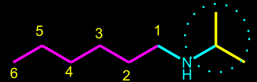
N -izopropil-heksan-1-amin
