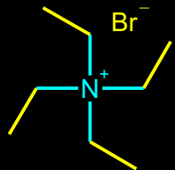
TETRAETIL-AMONIJUM BROMID
