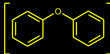
DIFENIL-ETAR
