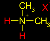
DIMETIL-AMONIUM JON
