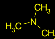
TRIMETIL-AMIN
