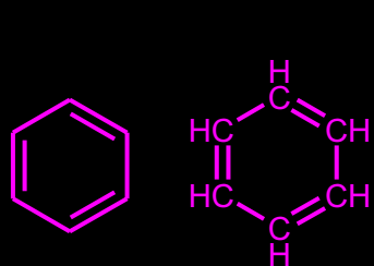
BENZEN
