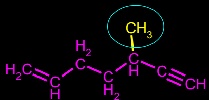
5-METIL-HEPT-1-EN-6-IN
