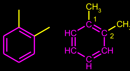
o-KSILEN
