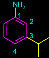
3-izo-PROPIL-ANILIN (3-izo-PROPIL-BENZEN-AMIN)
