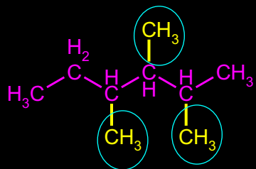
2,3,4-TRIMETIL-HEKSAN
