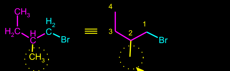
2-METIL-1-BROM-BUTAN
