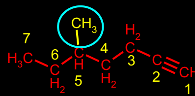
5-METIL-HEPT-1-IN
