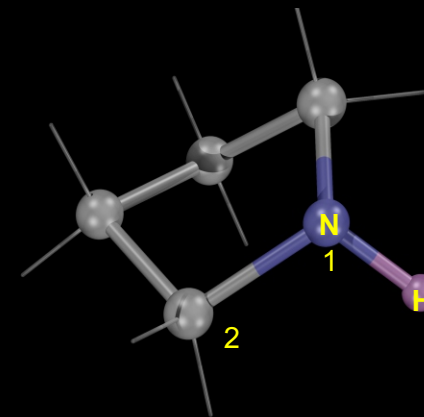
PIROLIDIN
