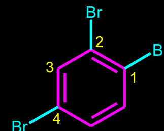
1,2,4-Tribrom-benzen
