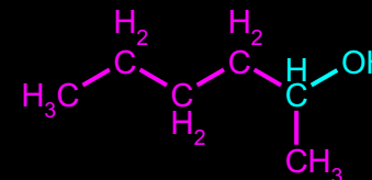
Hexan-2-ol
