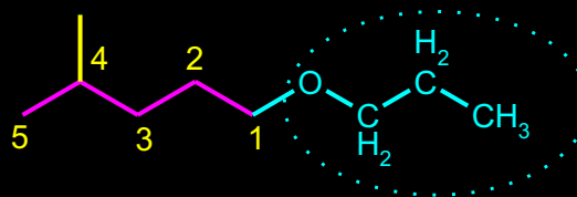
4-Metil-1-propoksi-pentan
