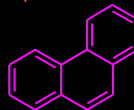
FENANTREN
