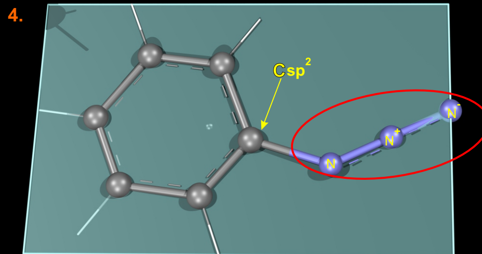
AZIDO-BENZEN
