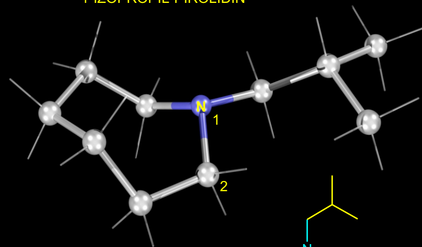
1-IZOPROPIL-PIROLIDIN
