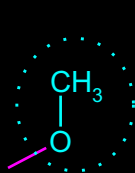
METOKSI
