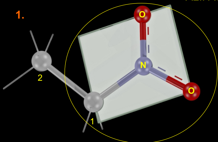
NITRO-ETAN
