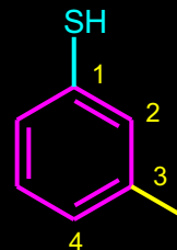
3-METIL-BENZENTIOL ILI 3-METIL-BENZEN-1-TIOL
