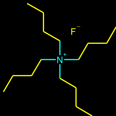
TETRABUTIL-AMONIJUM FLUORID
