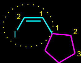
((Z)-2-Iodo-vinyl)-cyclopentane
