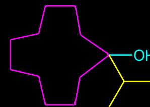
1-Izopropil- cikloundekanol
