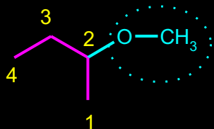
2-Metoksi-butan
